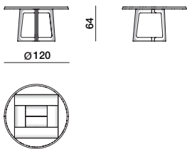
Tavolo lounge FTL12
