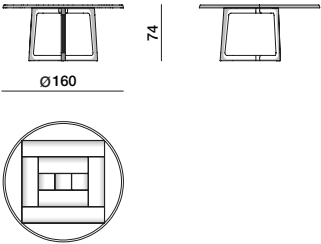
Tavolo tondo FTR16
